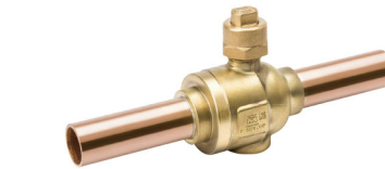
Valve à bille pour CO2 de type transcritique
